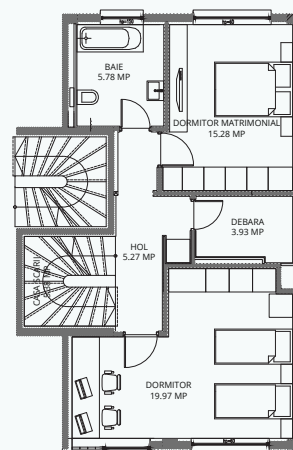
Etaj 1 ▲
