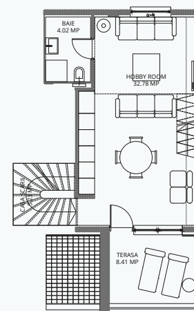
Etaj 2 ▲
